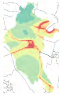
Conc. media annua - Settore: Altro
