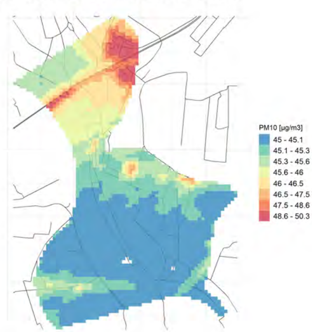
90.4° percentile della conc. media giornaliera di PM10
