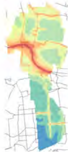
Conc. media annua - Settore: Altrc
