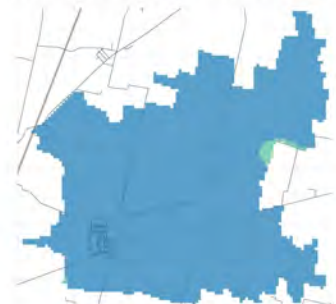
Concentrazione media centro abitato
