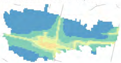
Conc. media annua - Settore: Trasporti
