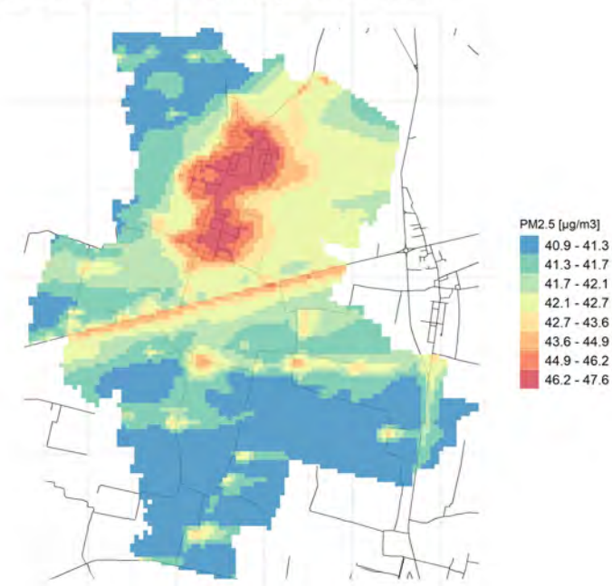
90.4° percentile della conc. media giornaliera di PM2.5
