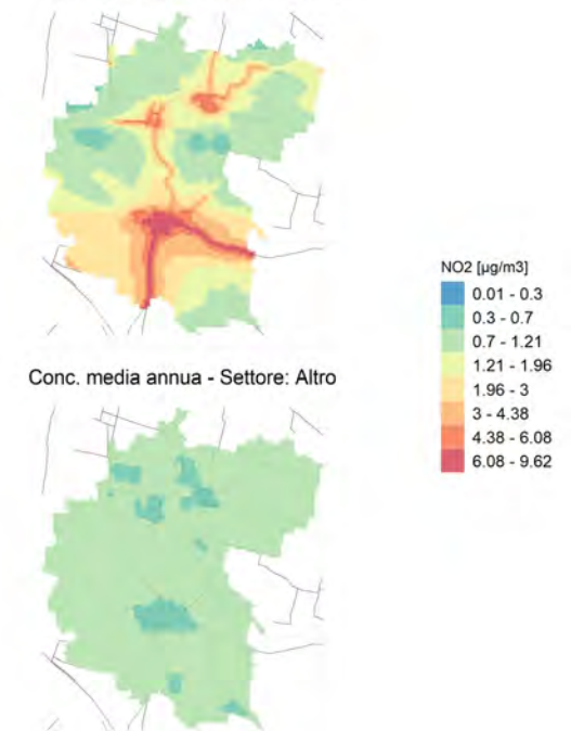
Conc. media annua - Settore: Trasporti
