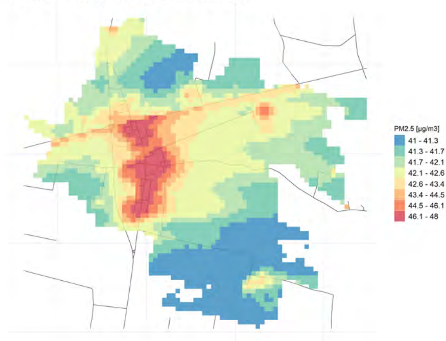
90.4° percentile della conc. media giornaliera di PM2.5
