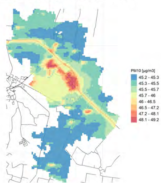
90.4° percentile della conc. media giornaliera di PM10
