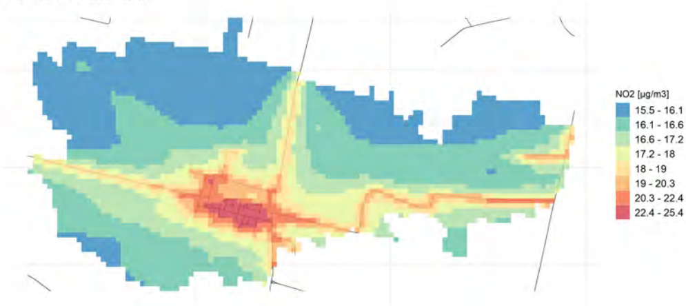
Conc. media annua NO2
