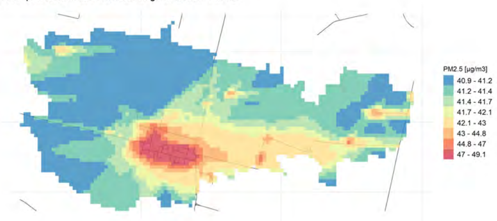
90.4° percentile della conc. media giornaliera di PM2.5
