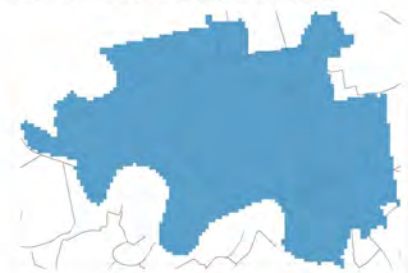
Conc. media annua - Settore: Industriale
