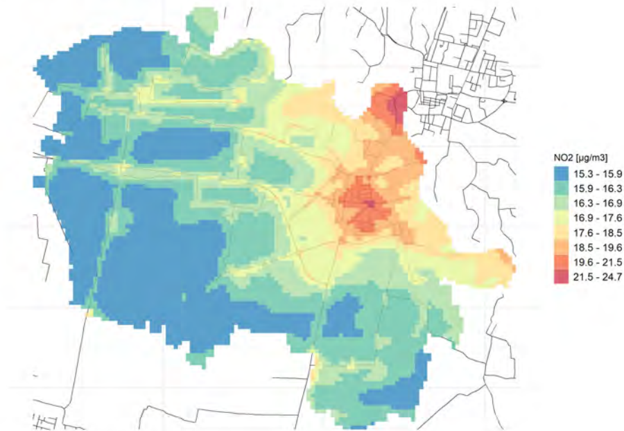
Conc. media annua NO2
