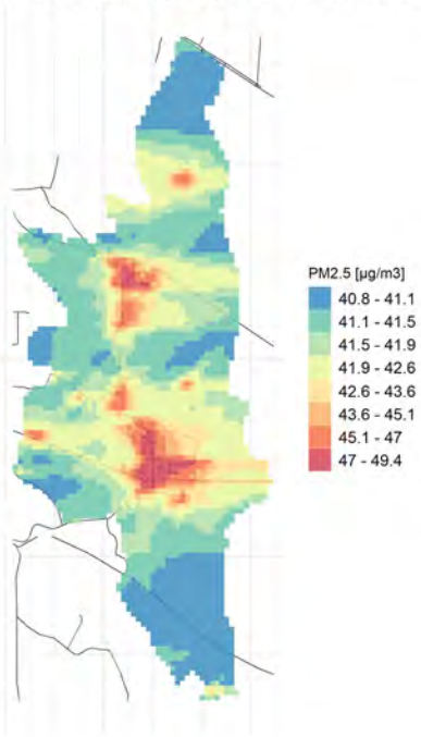
90.4° percentile della conc. media giornaliera di PM2.5
