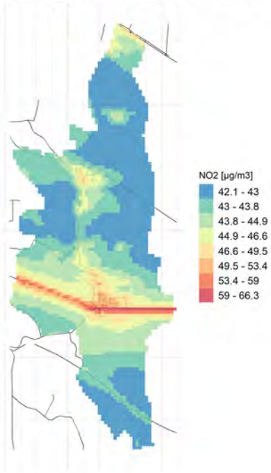
Massima concentrazione giornaliera di NO2
