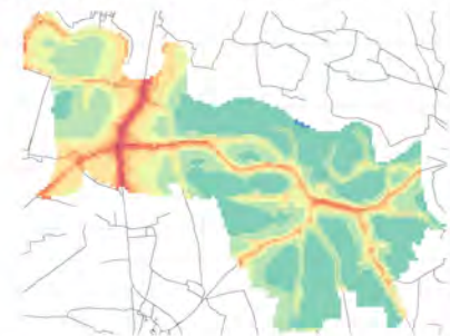
Conc. media annua - Settore: Trasporti
