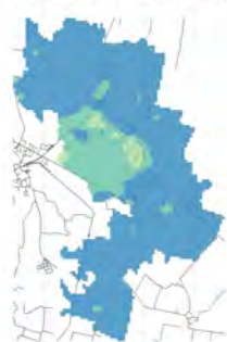
Conc. media annua - Settore: Industria
