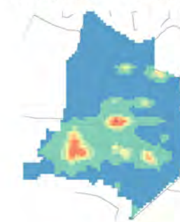
Concentrazione media centro abitato
