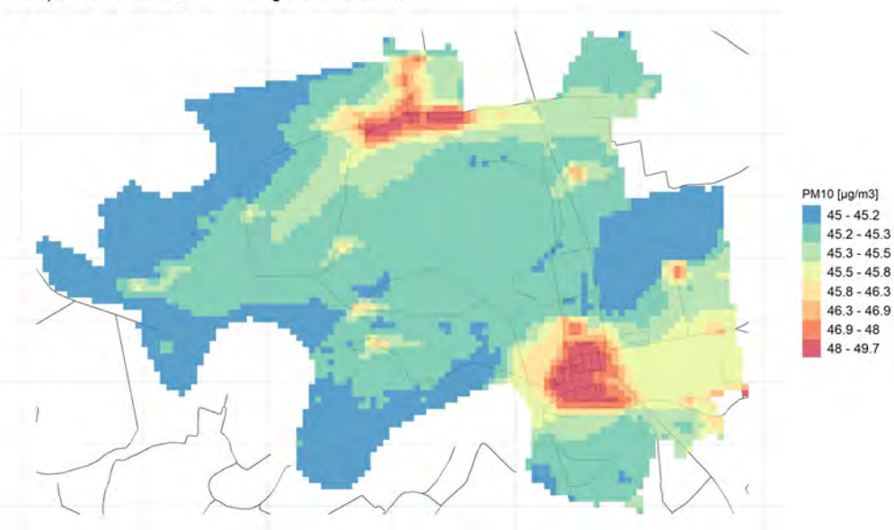
90.4° percentile della conc. media giornaliera di PM10
