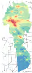
Conc. media annua - Settore: Indu
