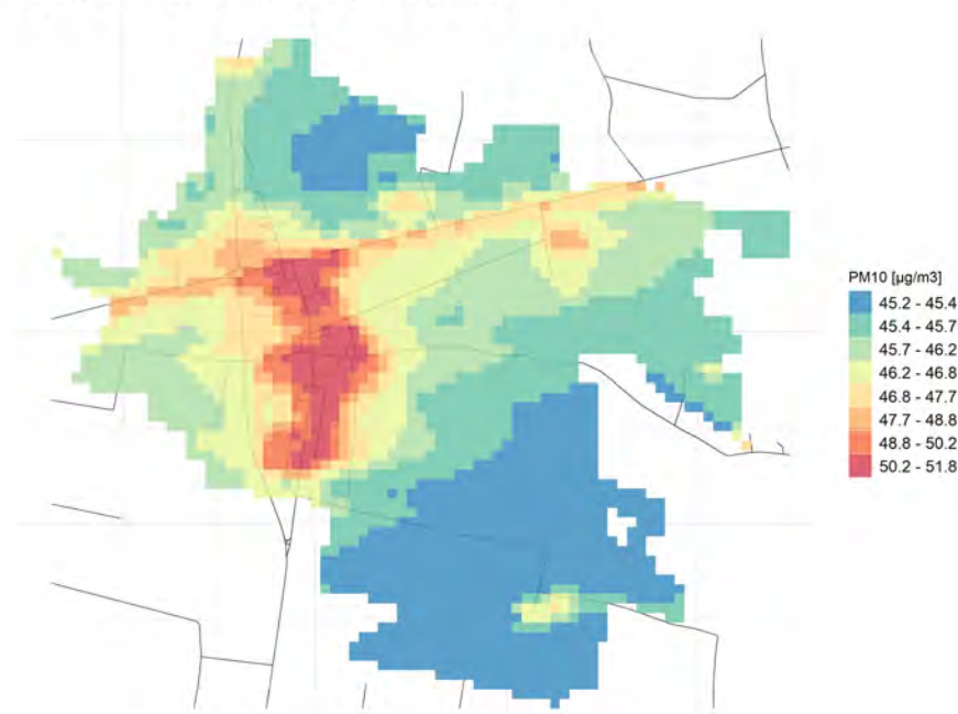
90.4° percentile della conc. media giornaliera di PM10
