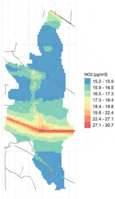
Conc. media annua NO2
