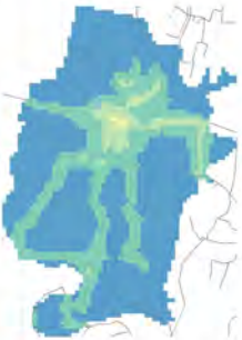
Conc. media annua - Settore: Altro
