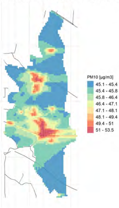
90.4° percentile della conc. media giornaliera di PM10
