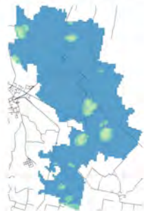
Concentrazione media centro abitato
