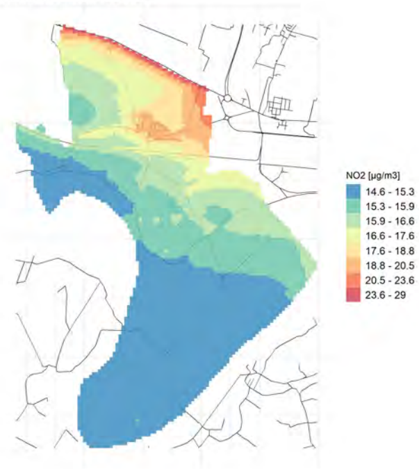
Conc. media annua NO2
