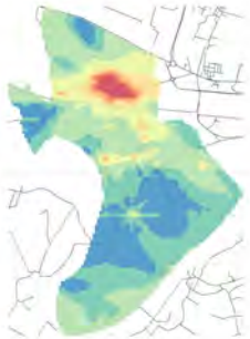
Conc. media annua - Settore: Industriale
