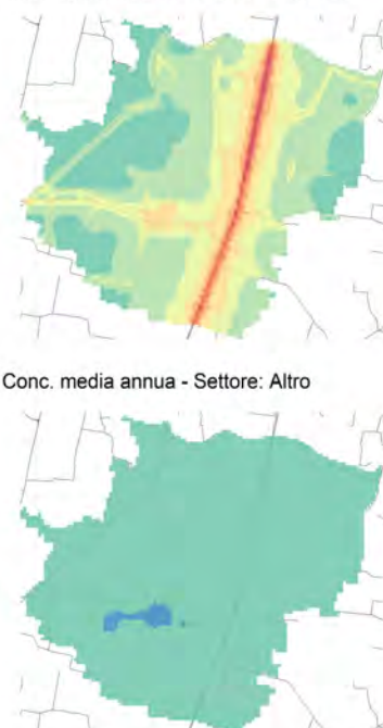
Conc. media annua - Settore: Trasporti
