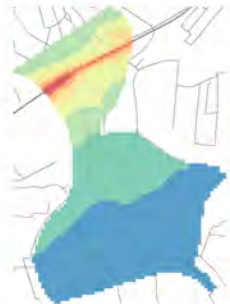
Conc. media annua - Settore: Altro
