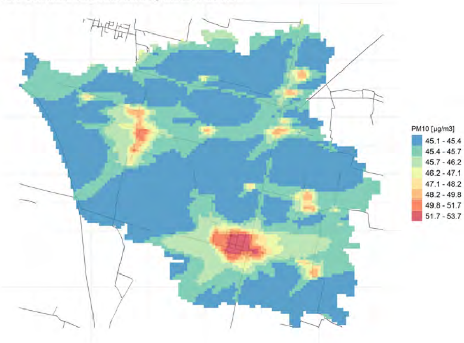
90.4° percentile della conc. media giornaliera di PM10
