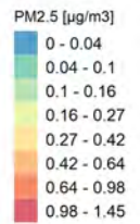
Conc. media annua - Settore: Altro
