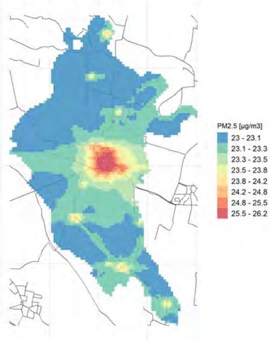
90.4° percentile della conc. media giornaliera di PM2.5
