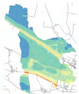
Conc. media annua - Settore: Altro
