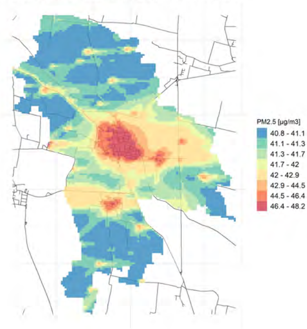
90.4° percentile della conc. media giornaliera di PM2.5
