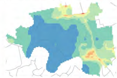
Conc. media annua - Settore: Trasporti
