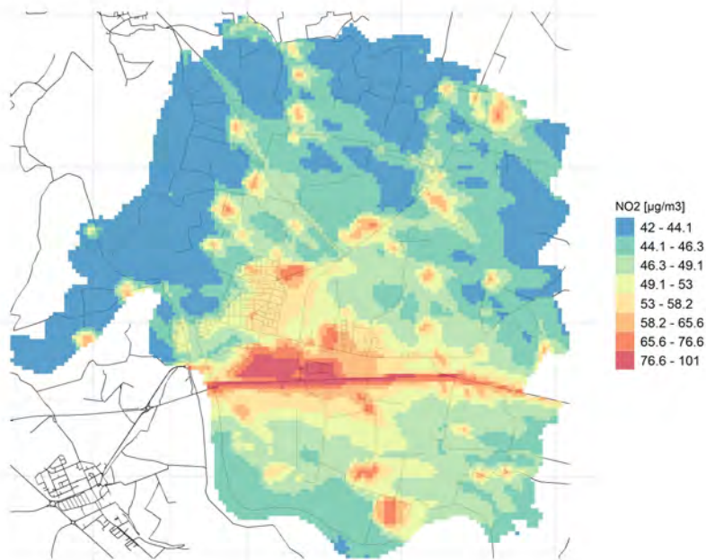
Massima concentrazione giornaliera di NO2
