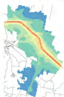
Conc. media annua - Settore: Altro
