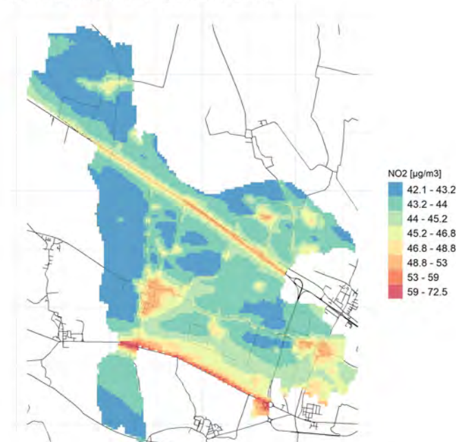
Massima concentrazione giornaliera di NO2
