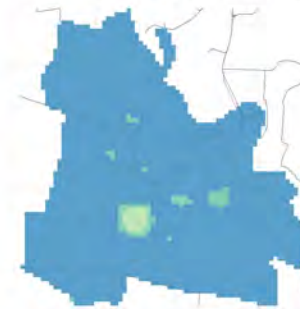
Concentrazione media centro abitato
