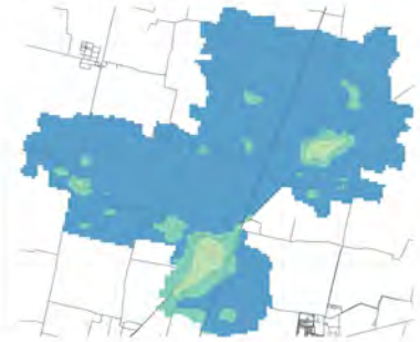
Conc. media annua - Settore: Industriale
