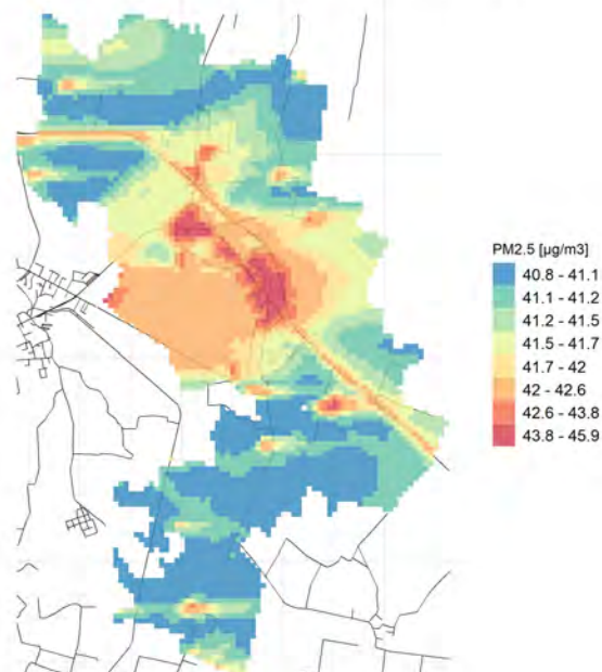
90.4° percentile della conc. media giornaliera di PM2.5
