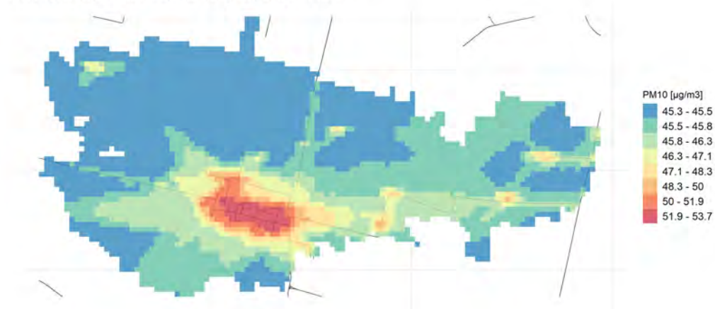
90.4° percentile della conc. media giornaliera di PM10
