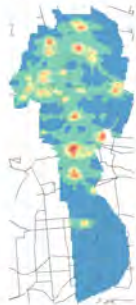
Concentrazione media centro abitato
