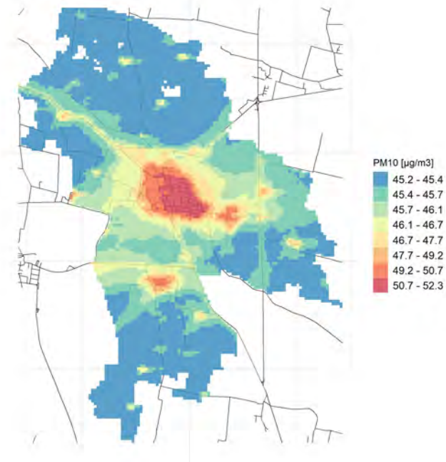
90.4° percentile della conc. media giornaliera di PM10
