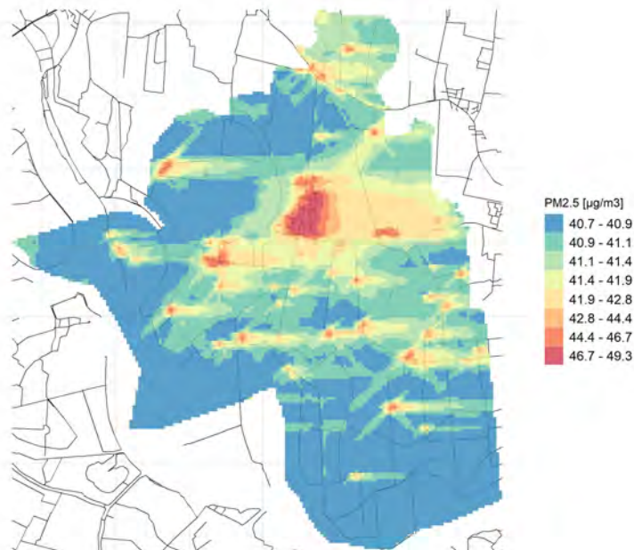
90.4° percentile della conc. media giornaliera di PM2.5
