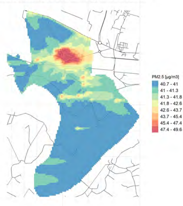
90.4° percentile della conc. media giornaliera di PM2.5
