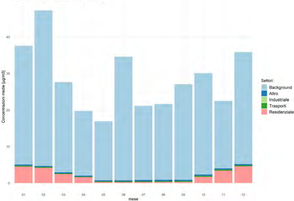
Concentrazione media centro abitato
