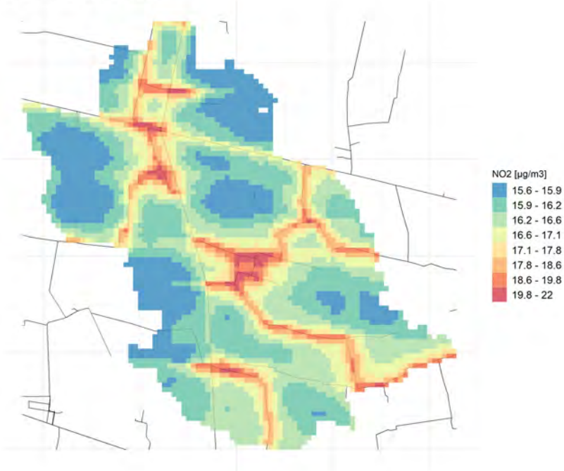
Massima concentrazione giornaliera di NO2
