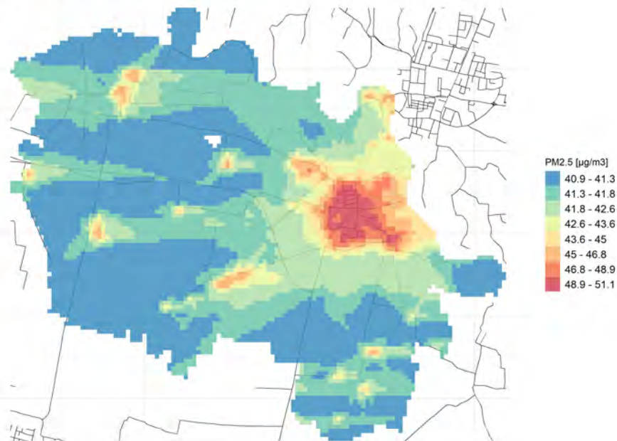
90.4° percentile della conc. media giornaliera di PM2.5
