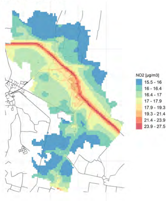
Conc. media annua NO2
