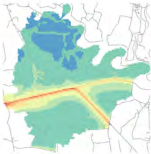
Conc. media annua - Settore: Altro
