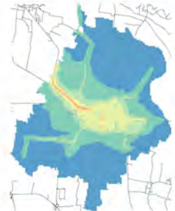
Conc. media annua - Settore: Altro
