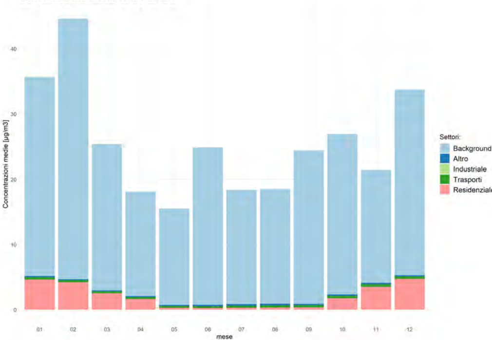
Concentrazione media centro abitato
