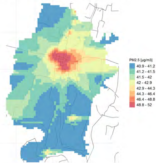
90.° percentile della conc. media giornaliera di PM2.5
