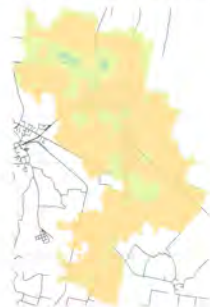
Conc. media annua - Settore: Altro
