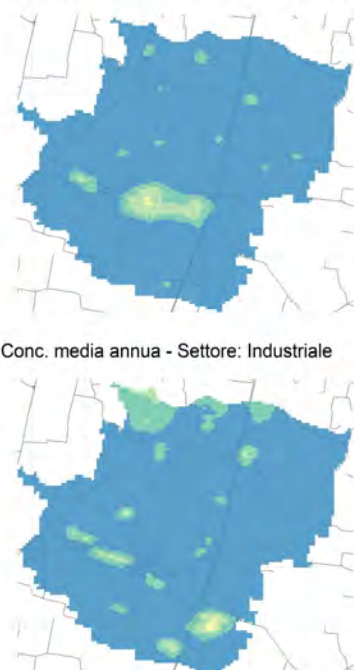
Conc. media annua - Settore: Residenziale
