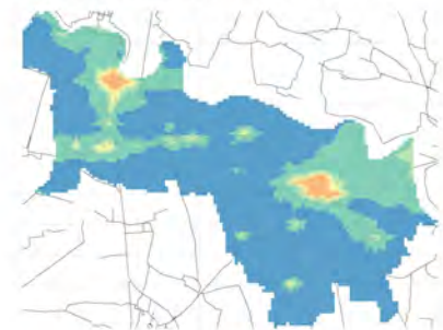
Conc. media annua - Settore: Residenziale
