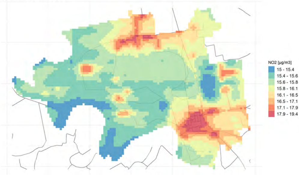
Conc. media annua NO2
