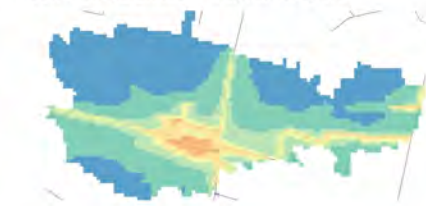
Conc. media annua - Settore: Trasporti
