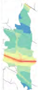
Conc. media annua - Settore: Altri
