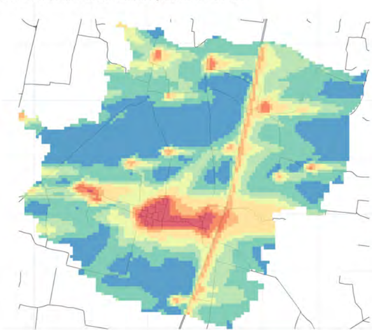
90.4° percentile della conc. media giornaliera di PM2.5
