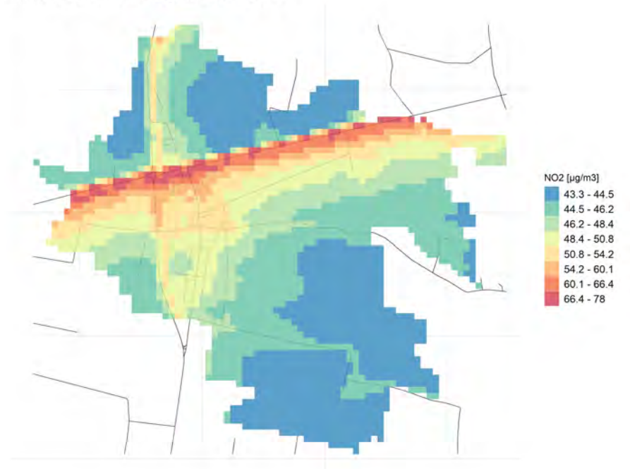
Massima concentrazione giornaliera di NO2
