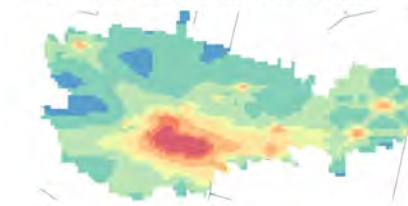
Conc. media annua - Settore: Residenziale
