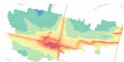
Conc. media annua - Settore: Trasporti
