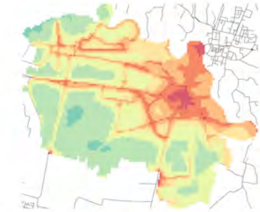
Conc. media annua - Settore: Altro
