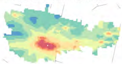
Conc. media annua - Settore: Residenziale
