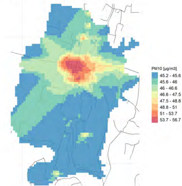
90.° percentile della conc. media giornaliera di PM10
