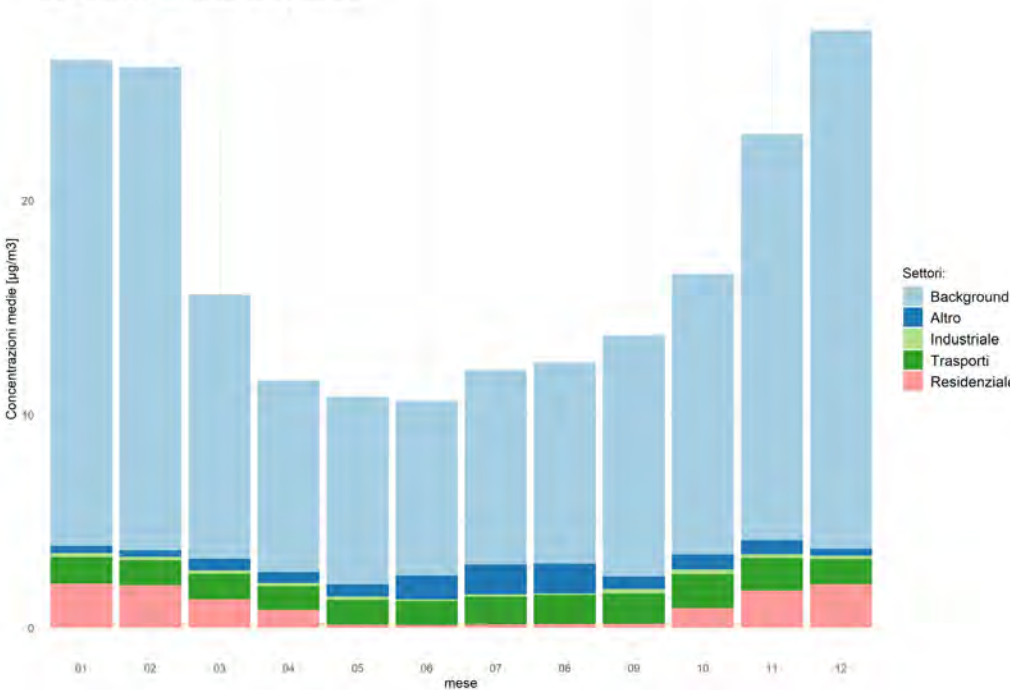
Concentrazione media centro abitato
