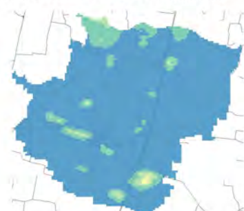
Conc. media annua - Settore: Industriale
