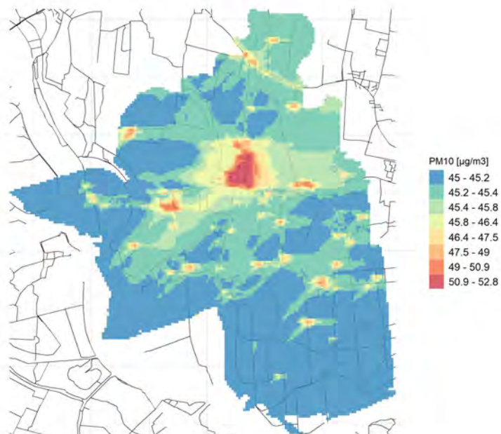
90.4° percentile della conc. media giornaliera di PM10
