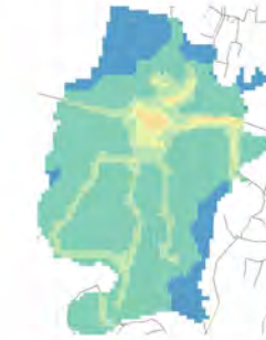
Conc. media annua - Settore: Altro
