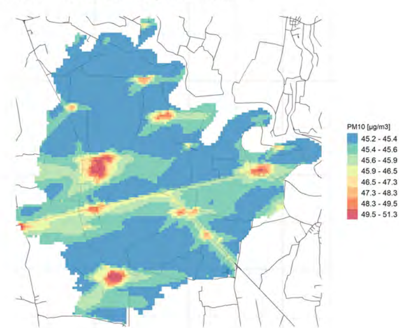
90.4° percentile della conc. media giornaliera di PM10
