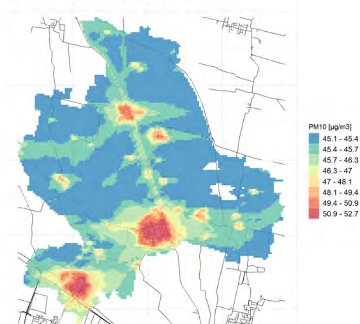
90.4° percentile della conc. media giornaliera di PM10
