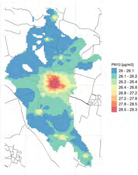
90.4° percentile della conc. media giornaliera di PM10
