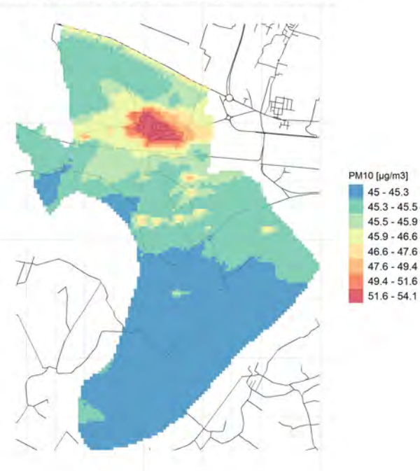
90.4° percentile della conc. media giornaliera di PM10
