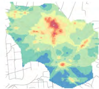
Conc. media annua - Settore: Industriale
