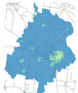
Conc. media annua - Settore: Industriale
