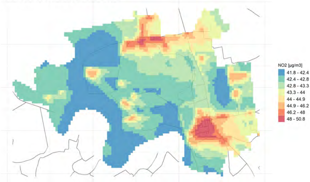
Massima concentrazione giornaliera di NO2
