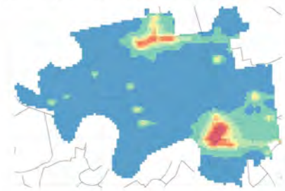
Conc. media annua - Settore: Residenziale
