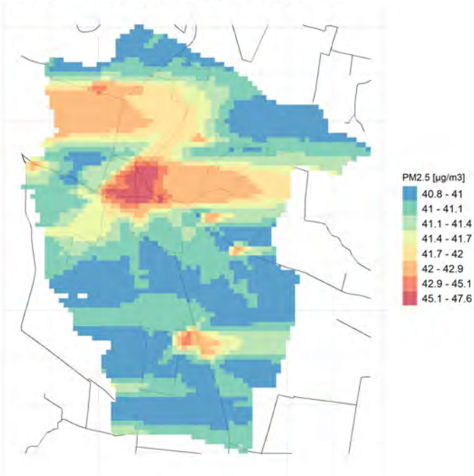
90.4° percentile della conc. media giornaliera di PM2.5
