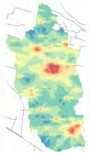
Conc. media annua - Settore: Industri
