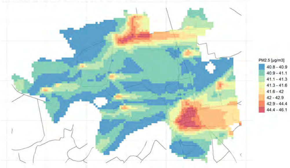
90.4° percentile della conc. media giornaliera di PM2.5
