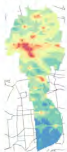
Conc. media annua - Settore: Indu
