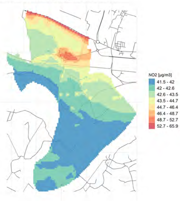
Massima concentrazione giornaliera di NO2
