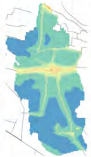
Conc. media annua - Settore: Altro
