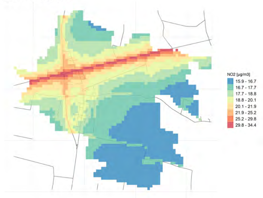
Conc. media annua NO2
