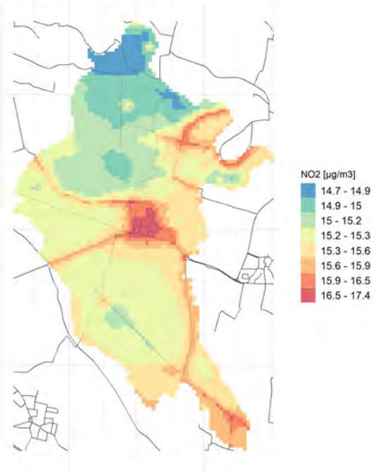
Massima concentrazione giornaliera di NO2
