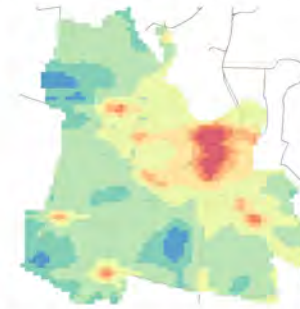
Conc. media annua - Settore: Industriale
