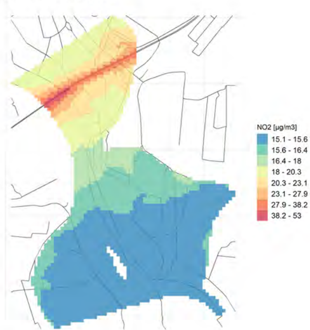
Conc. media annua NO2
