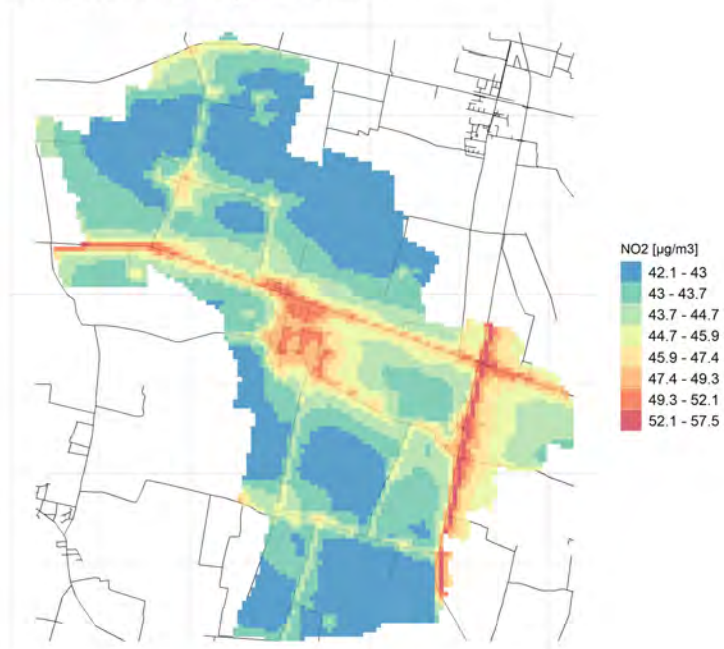
Massima concentrazione giornaliera di NO2
