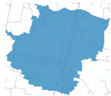
Concentrazione media centro abitato
