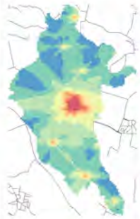
Conc. media annua - Settore: Industri
