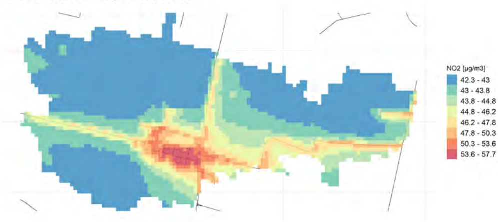
Massima concentrazione giornaliera di NO2
