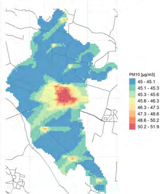
90.4° percentile della conc. media giornaliera di PM10
