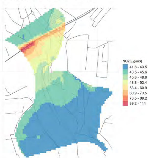
Massima concentrazione giornaliera di NO2
